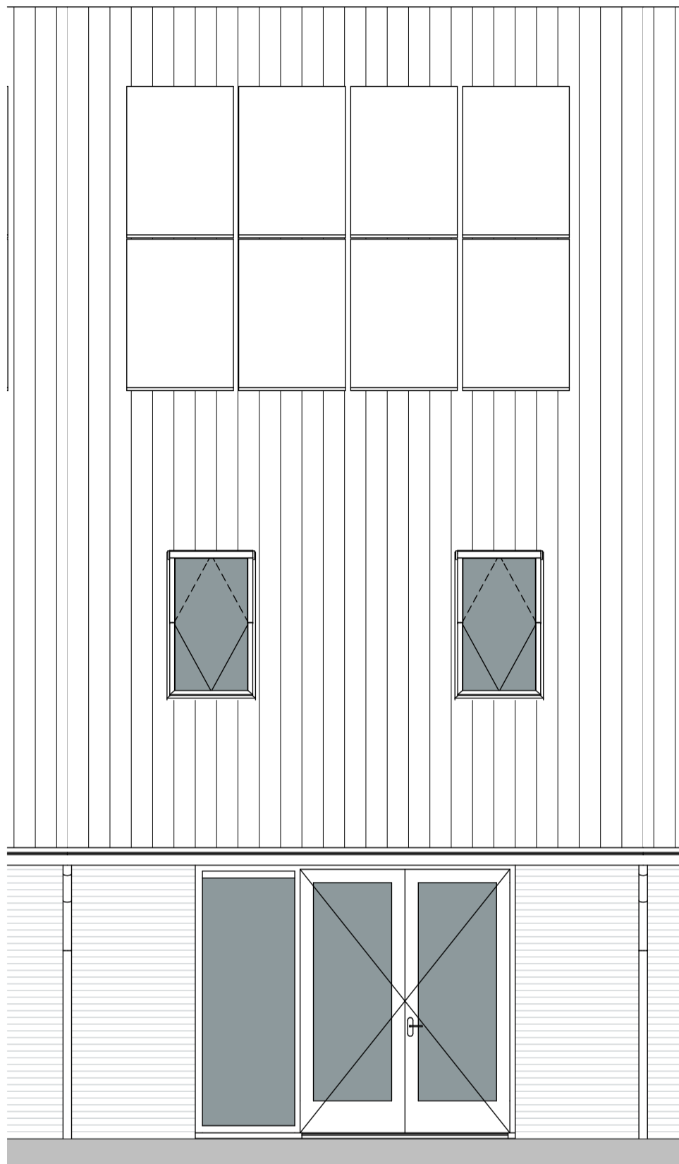
Achtergevel
